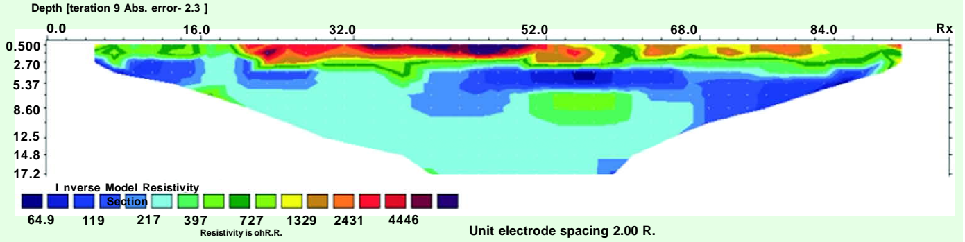
आकृति-1 (सी) रेजिस्टिविटी इमेजिंग सिस्टम के उपयोग से एसएसबी मैदान, श्रीनगर में रेजिस्टिविटी विचलन
