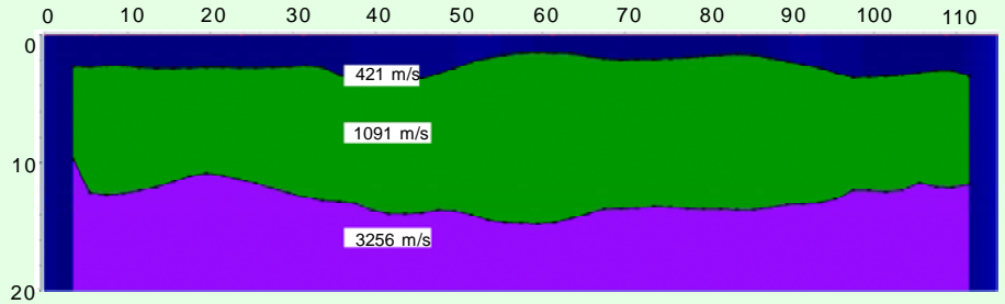
आकृति-1 (ए) रेफ्लेक्शन विधि के उपयोग से आईआईटी मैदान, श्रीनगर का पी वेव विचलन
